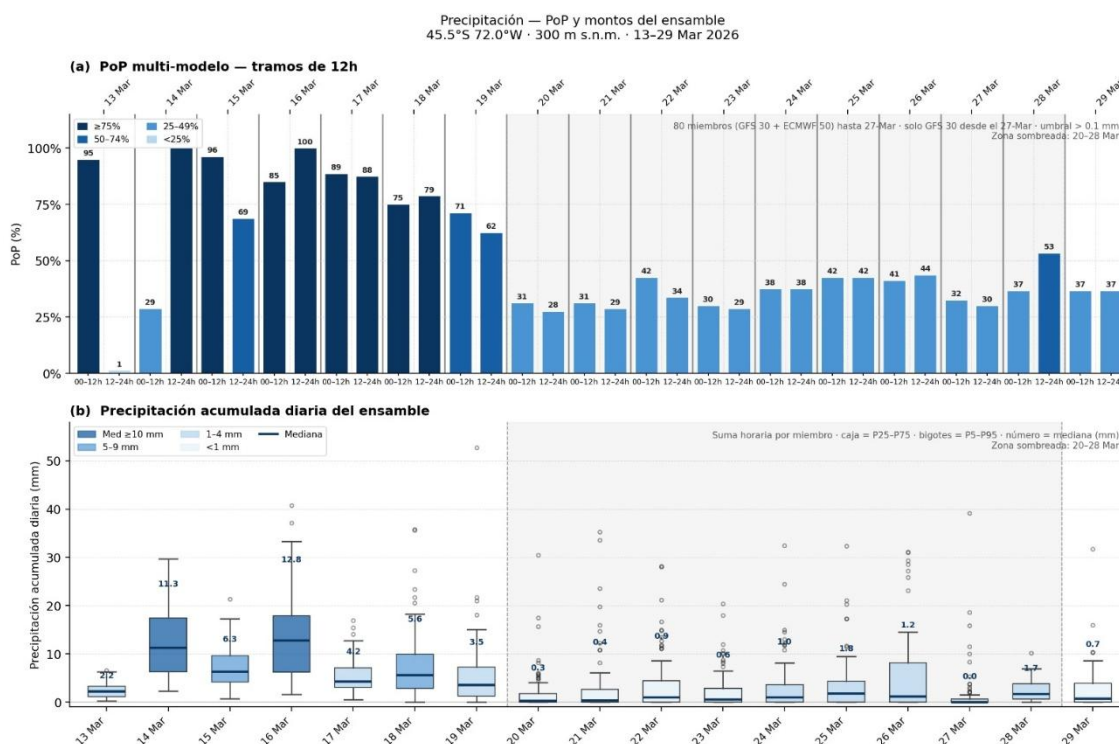
Figura 1. Proyección probabilística de precipitación (simulaciones de ensamble). Las barras muestran la probabilidad de lluvia basada en múltiples simulaciones de modelos. En general, la probabilidad de precipitación parece ser menor alrededor del 20–23 de marzo, con un ligero aumento entre el 24–26 de marzo. En la mayoría de los escenarios, las precipitaciones esperadas son ligeras (generalmente menores a 10 mm por día).
