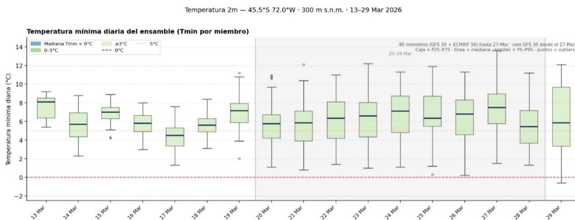
Figura 2. Proyección de temperaturas mínimas basada en simulaciones de ensamble. La mayoría de las simulaciones sugiere temperaturas mínimas diarias entre 4 °C y 8 °C durante el período del congreso, lo que indica mañanas y noches frescas, típicas del inicio del otoño en Patagonia.
